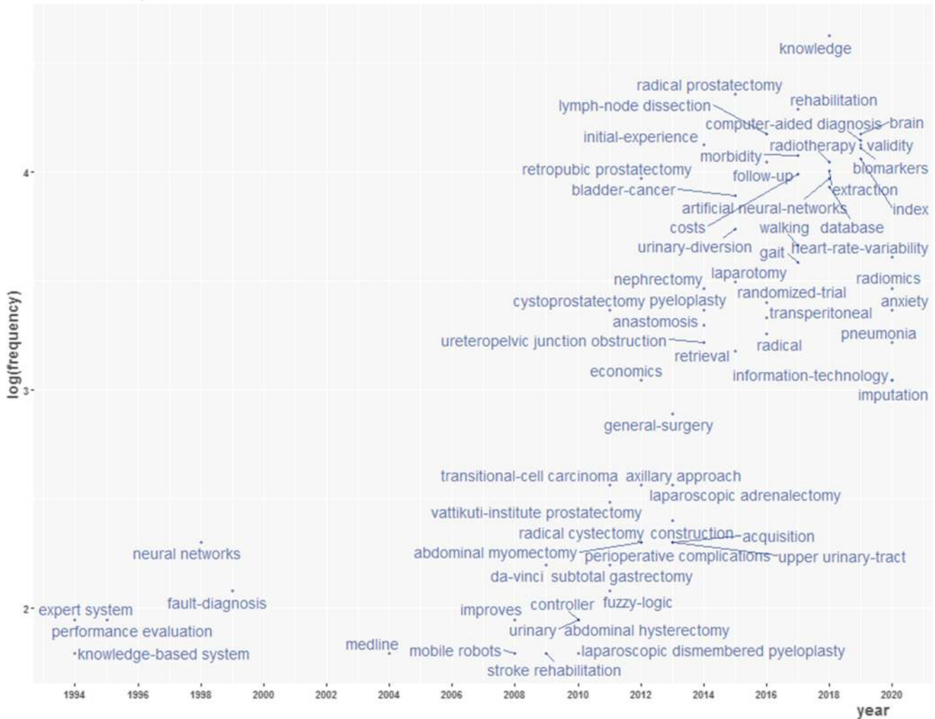
Fig. 4 Trend topics
