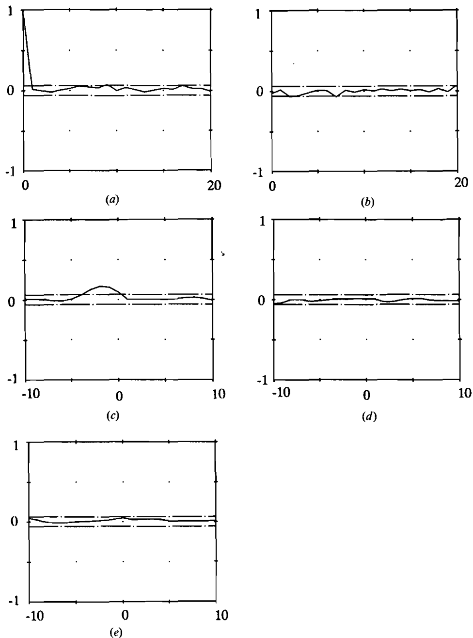
Figure 11. Correlation tests (Example 2): (a) \Psi_{ee}(k) ; (b) \Psi_{e(eu)}(k) ; (c) \Psi_{ue}(k) ; (d) \Psi_{uz_1}(k) ; (e) \Psi_{uz_2}(k) ; — · — 95% confidence band.
