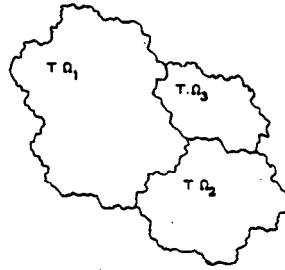
L'« échange de morceaux » T défini sur \Omega par : Tx = x + \xi (modulo Z^2 ).
