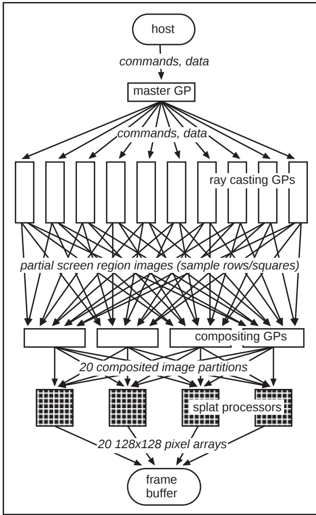
Fig. 1. VOL2 visualization pipeline.
