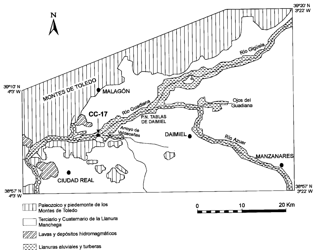
Figura 2. Esquema morfogeológico de la Cuenca Alta del Guadiana (simplificada de Pérez González, 1996) y localización del sondeo CC-17 Morpho-geological scheme of the High Basin of the river Guadiana (simplified from Pérez González, 1996) and location of core CC-17
