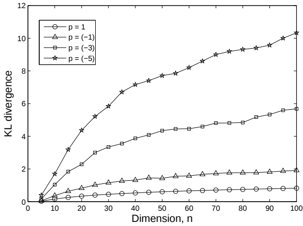
(b) CKF
