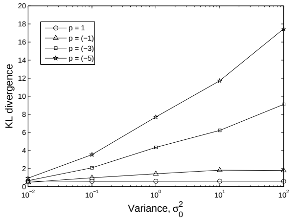
(b) CKF
