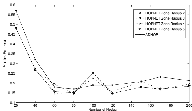
Fig. 8. Link Failures
