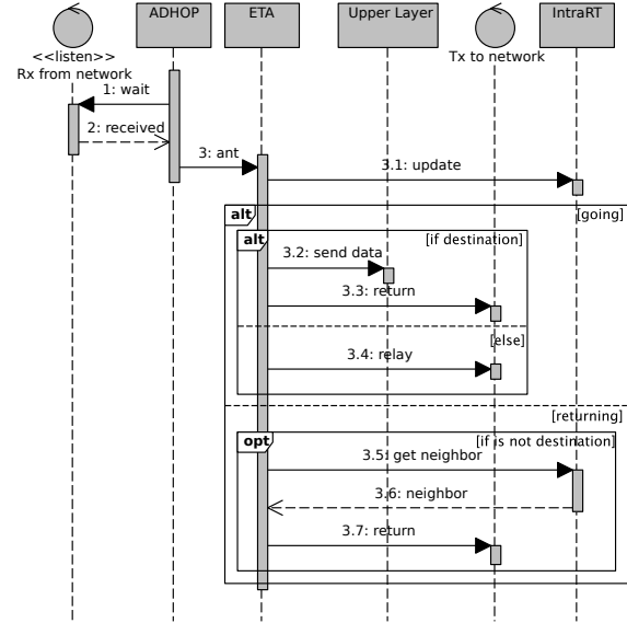
Fig. 4. ETA Rx
