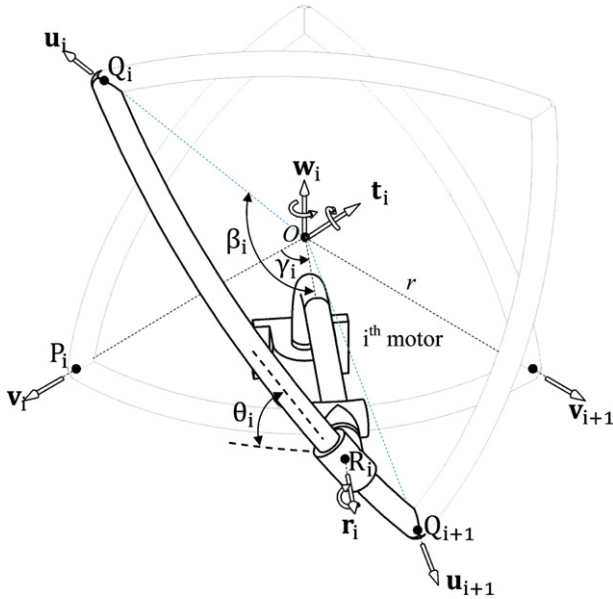
Fig. 3. Parameters description of ith leg.
